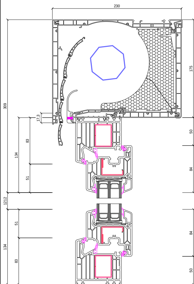
Presjek S1, M 5:1
